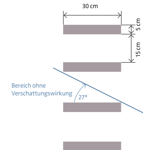
Schema horizontale Verschattungslamellen
