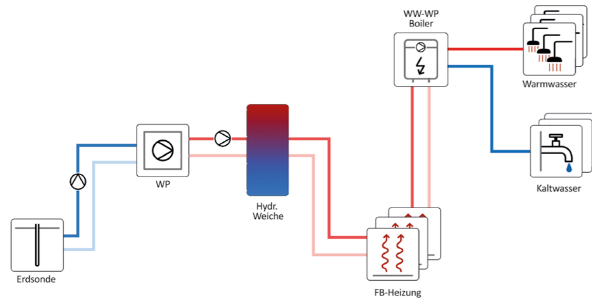
Einbindung der dezentralen Wärmepumpen-Boiler in den Heizkreis
