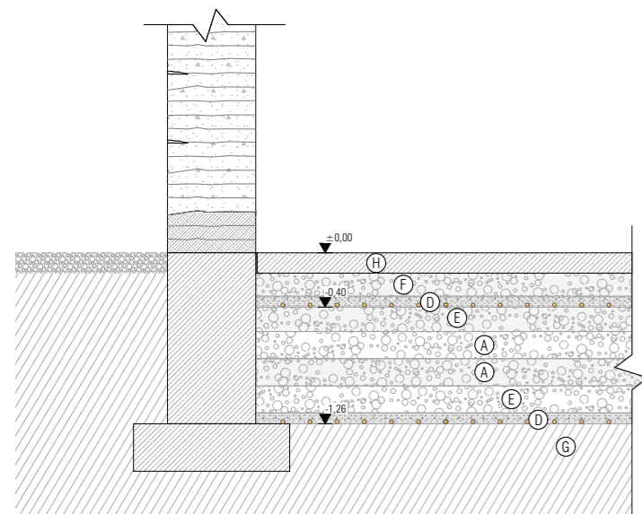
Detailschnitt Systemaufbau des Hallenbodens mit Anschluss an Stampflehmwand mit Sockel Stampfbeton
