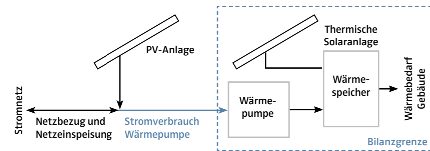
Messbilanz Wärmepumpe
