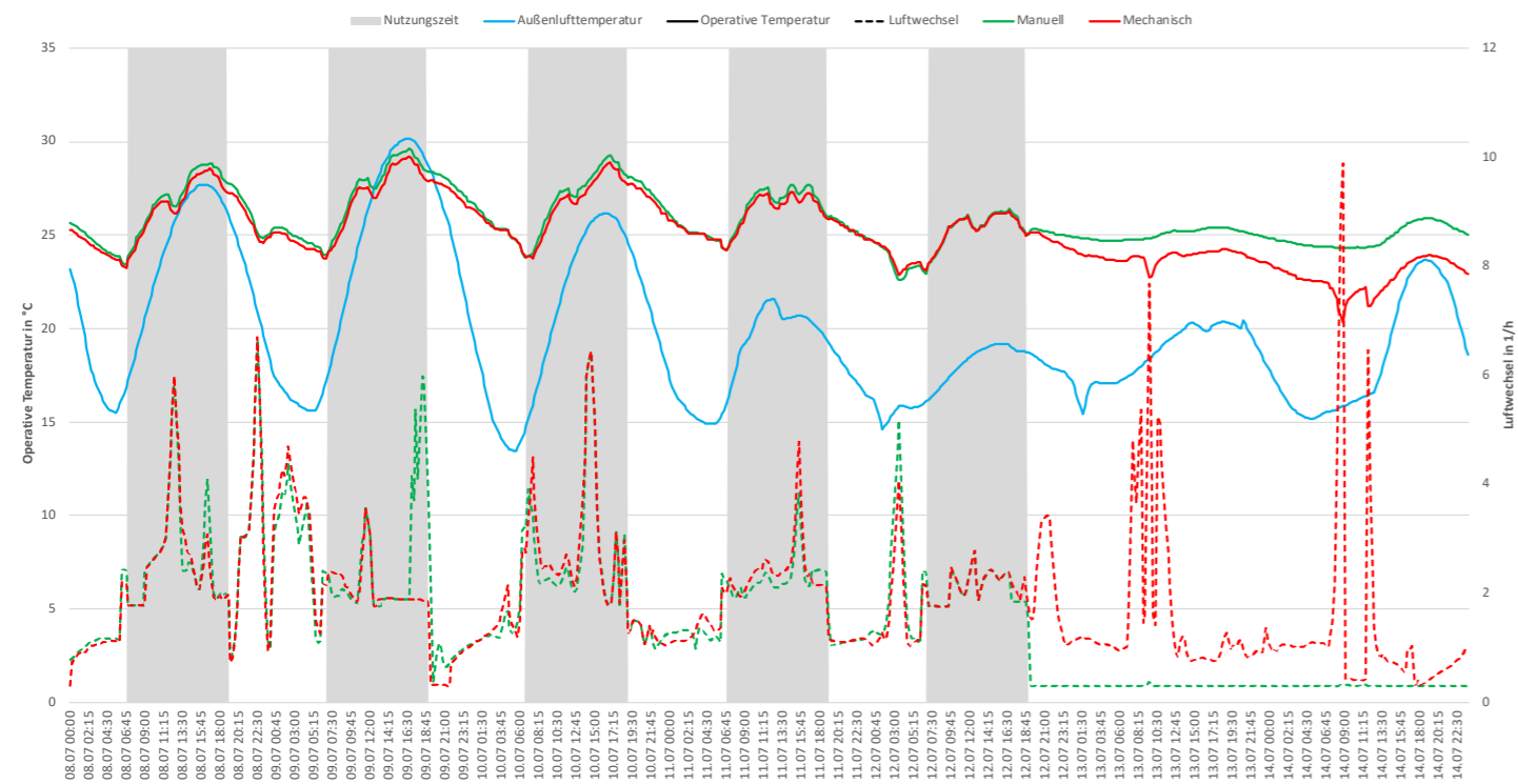
Operative Innenraumtemperatur und Luftwechselrate, Kalenderwoche 28
