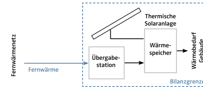
Messbilanz Fernwärme
